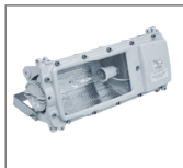
II 2G Ex de IIB T4-T3; II 2D Ex tD A21 T145°C-210°C; IP 66; HST/HIT; Kl. Ochr. I
